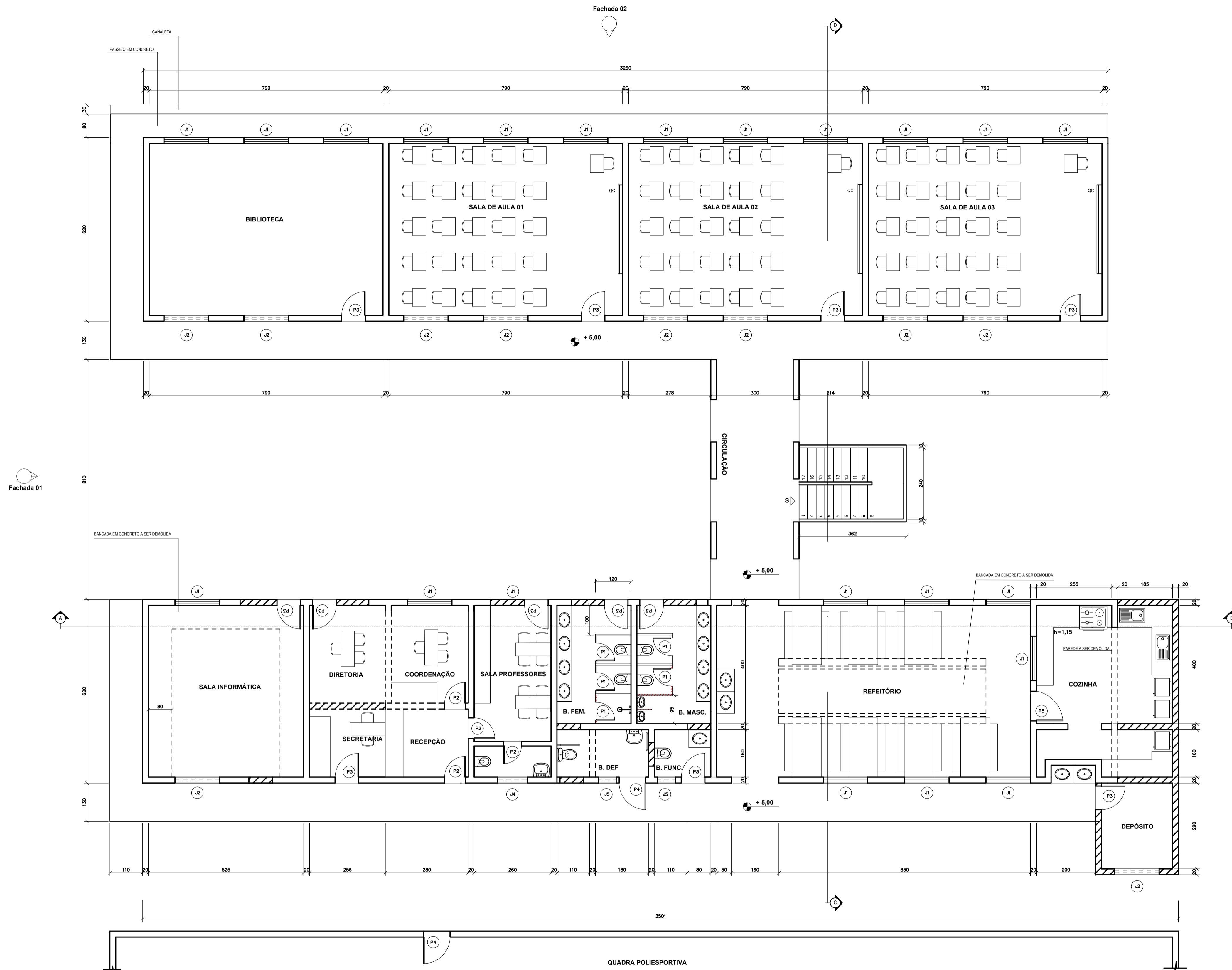
PLANTA BAIXA TÉRREO ESCALA: 1/75 MEDIDAS EM CENTÍMETROS, EXCETO INDICADAS
